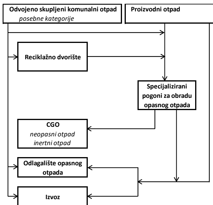
Slika 3.2.1/3 – Shema gospodarenja opasnim otpadom (izvor: IPZ Uniprojekt MCF)
