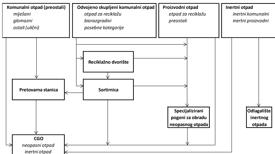
Slika 3.2.1/2 – Shema gospodarenja neopasnim i inertnim otpadom (izvor: IPZ Uniprojekt MCF)
