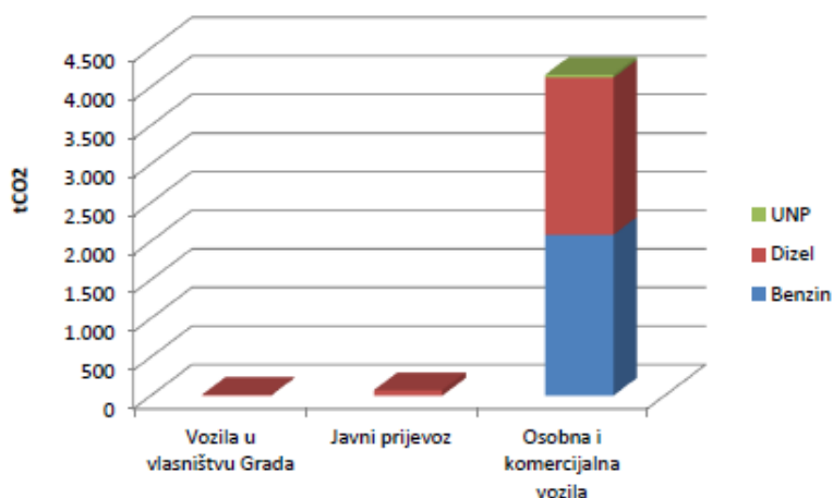
Slika 4-2 - Emisije CO 2 prometnog sektora Grada Belišća
