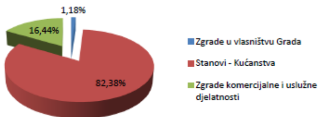
Slika 5-3 - Udio pojedinog podsektora u ukupnom kontrolnom inventaru emisija CO 2 sektora zgradarstva za 2020. godinu
