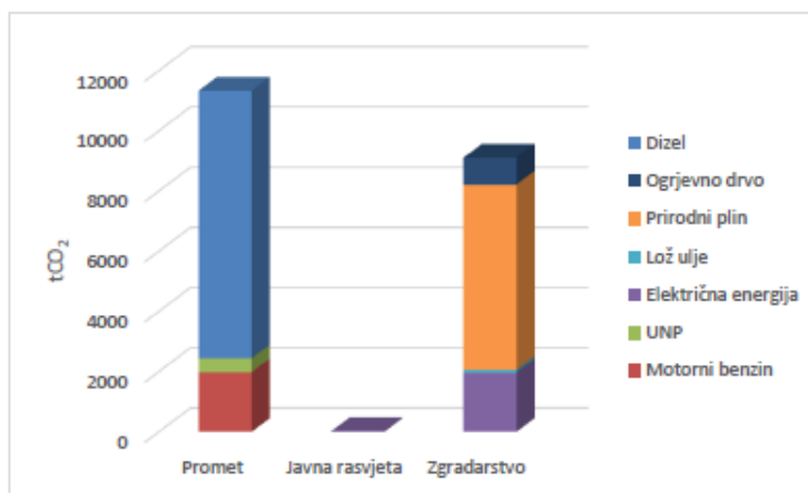
Slika 5-10 - Prikaz Kontrolnog inventara emisija CO 2 po sektorima i energentima u 2020. godini
