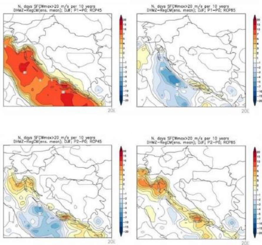
Slika 8-3 Promjena srednjeg broja dana s maksimalnom brzinom vjetra većim ili jednakom od 20 m/s, u odnosu na referentno razdoblje 1971. – 2000. Gore: za razdoblje 2011. – 2040. godine; dolje: za razdoblje 2041. – 2070. godine; lijevo: scenarij RCP4.5; desno: scenarij RCP8.5. Mjerna jedinica: broj događaja u 10 godina. Sezona: zima.
