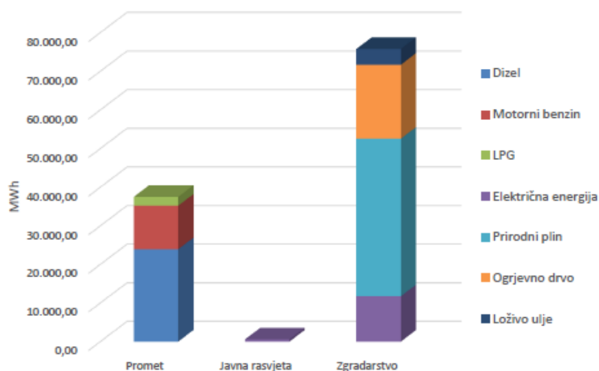
Slika 4-3 Struktura energetske potrošnje po energentu u 2009. godini
