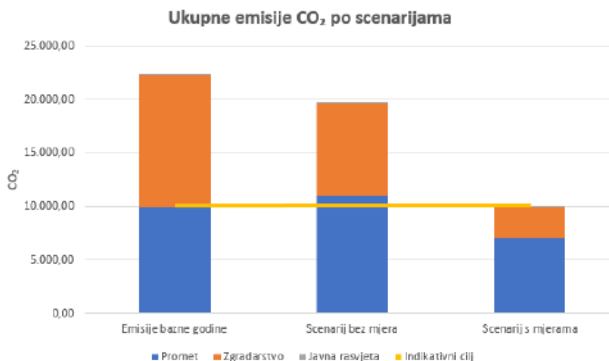
Slika 12-2 - Ukupne projekcije emisije CO 2 po scenarijima
