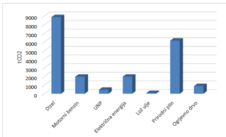
Slika 5-9 - Kontrolni inventar emisija CO 2 po energentima u 2020. godini
