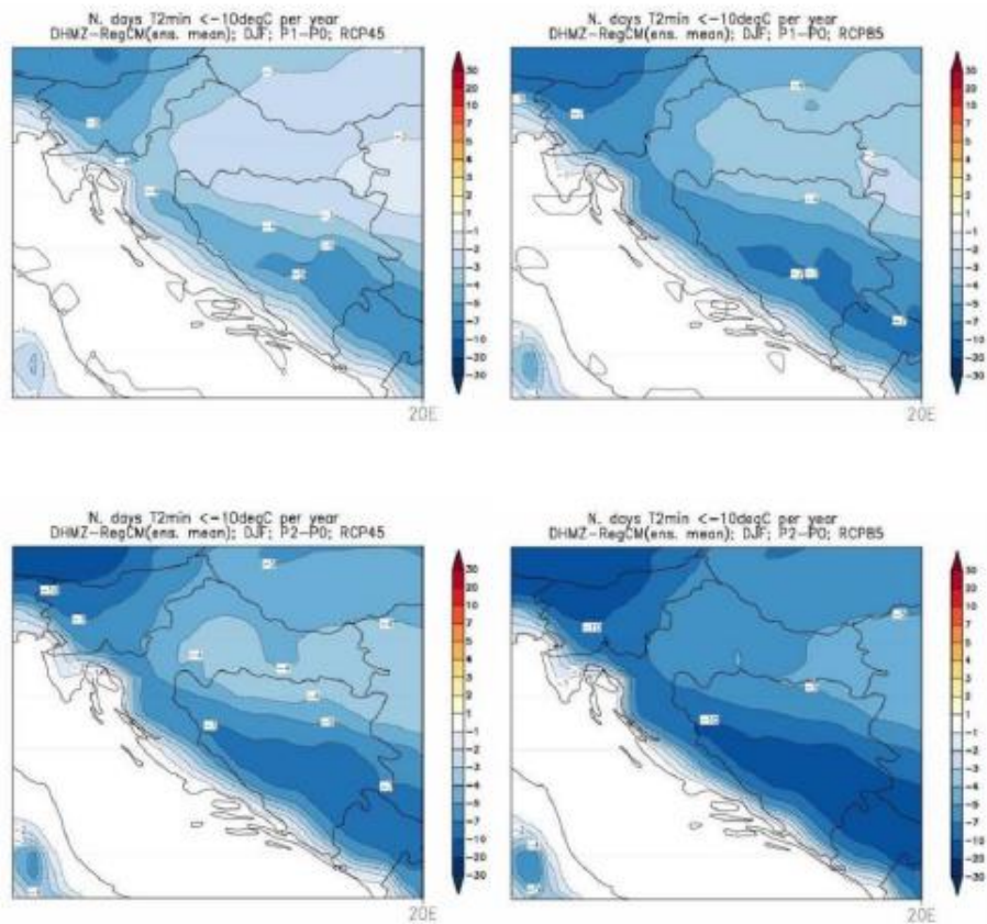
Slika 8-4 Promjena srednjeg broja ledenih dana (dan kad je minimalna temperatura manja ili jednaka -10^{\circ}\text{C} , u odnosu na referentno razdoblje 1971. – 2000. Gore: za razdoblje 2011. – 2040. godine; dolje: za razdoblje 2041. – 2070. godine; lijevo: scenarij RCP4.5; desno: scenarij RCP8.5. Mjerna jedinica: broj događaja u godini. Sezona: zima.
