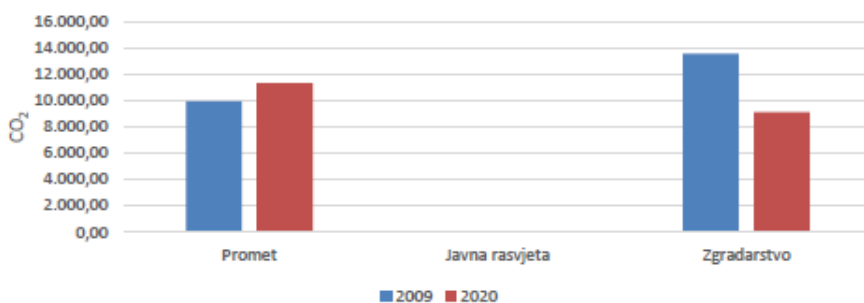
Slika 6-2 Usporedba Referentnog i Kontrolnog inventara emisija CO 2 po sektorima
