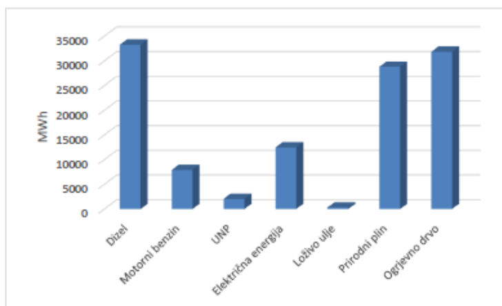
Slika 5-6 - Energetska potrošnja po energentu u 2020. godini
