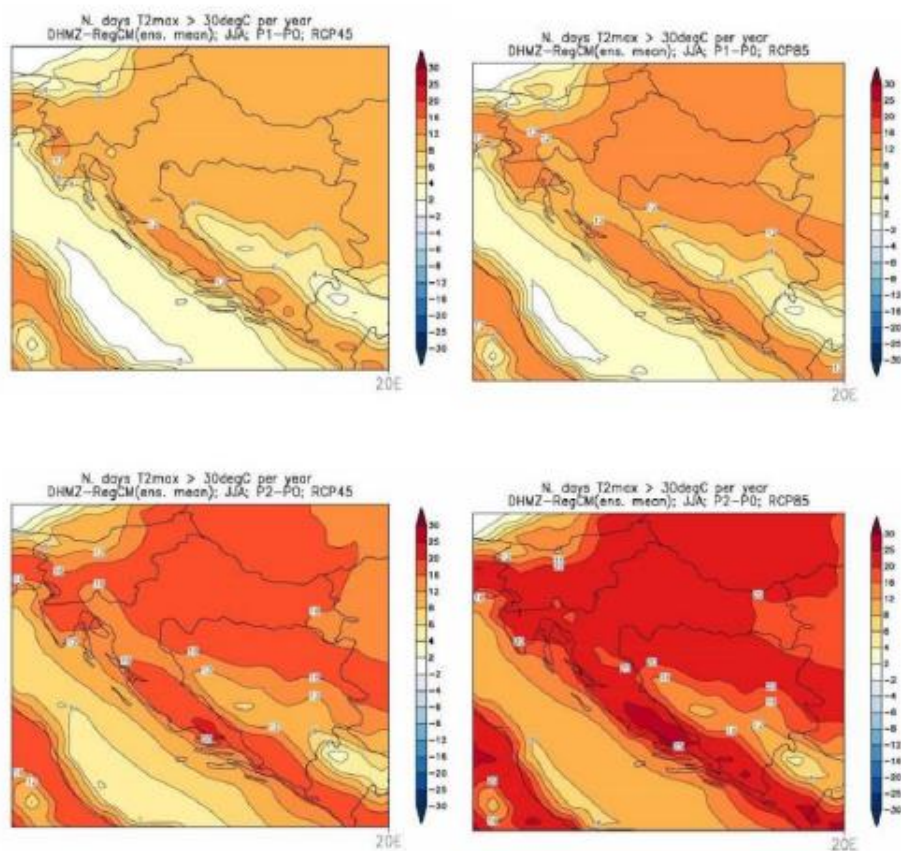
Slika 8-5. Promjena srednjeg broja vrućih dana (dan kad je maksimalna temperatura veća ili jednaka 30^{\circ}\text{C} ), u odnosu na referentno razdoblje 1971. – 2000. Gore: za razdoblje 2011. – 2040. godine; dolje: za razdoblje 2041. – 2070. godine; lijevo: scenarij RCP4.5; desno: scenarij RCP8.5. Mjerna jedinica: broj događaja u sezoni. Sezona: ljeto.
