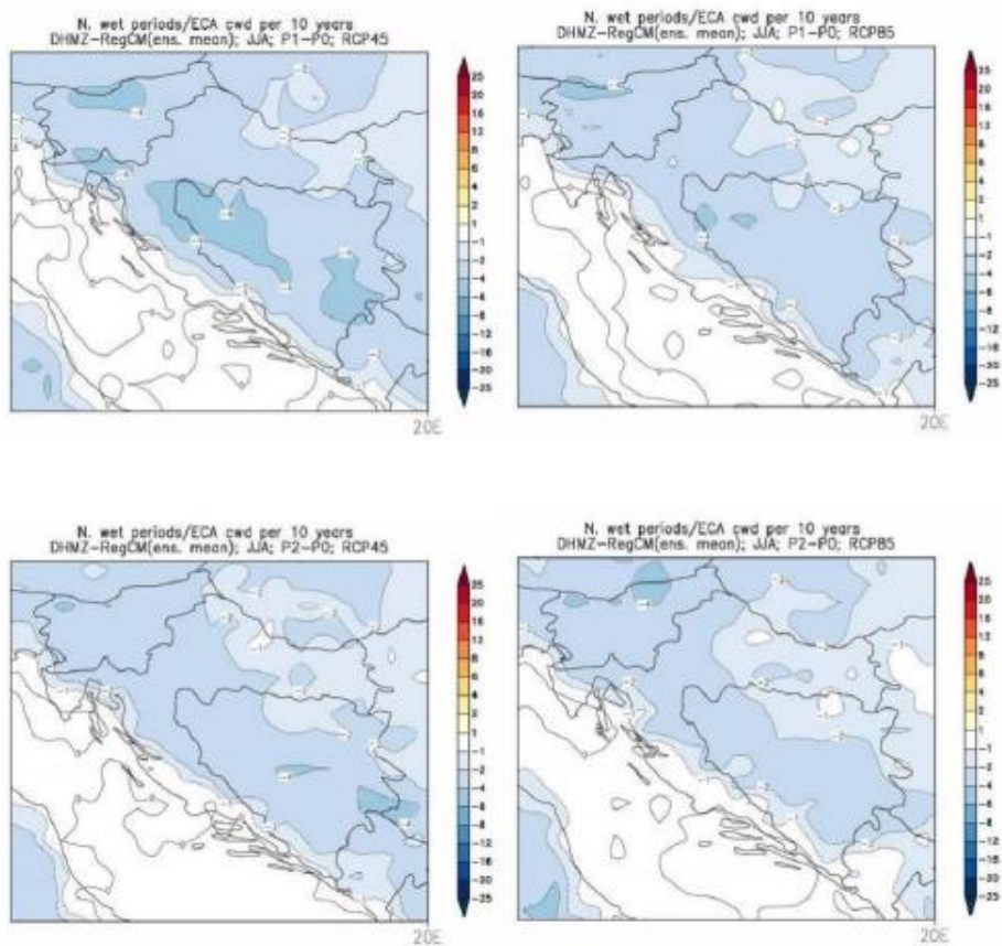
Slika 8-6. Promjena srednjeg broja kišnih razdoblja, u odnosu na referentno razdoblje 1971. – 2000. Gore: za razdoblje 2011. – 2040. godine; dolje: za razdoblje 2041. – 2070. godine; lijevo: scenarij RCP4.5; desno: scenarij RCP8.5. Mjerna jedinica: broj događaja u 10 godina. Sezona: ljeto.
