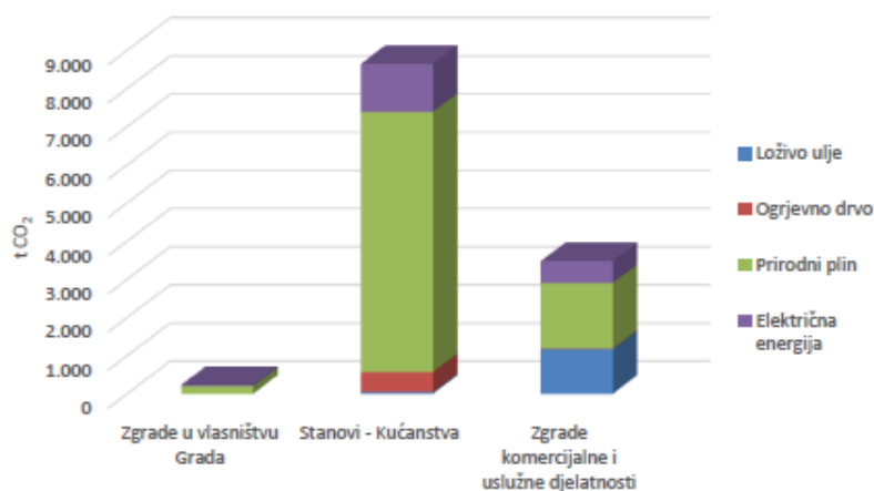
Slika 4-1 - Emisije CO 2 sektora zgradarstva Grada Belišća
