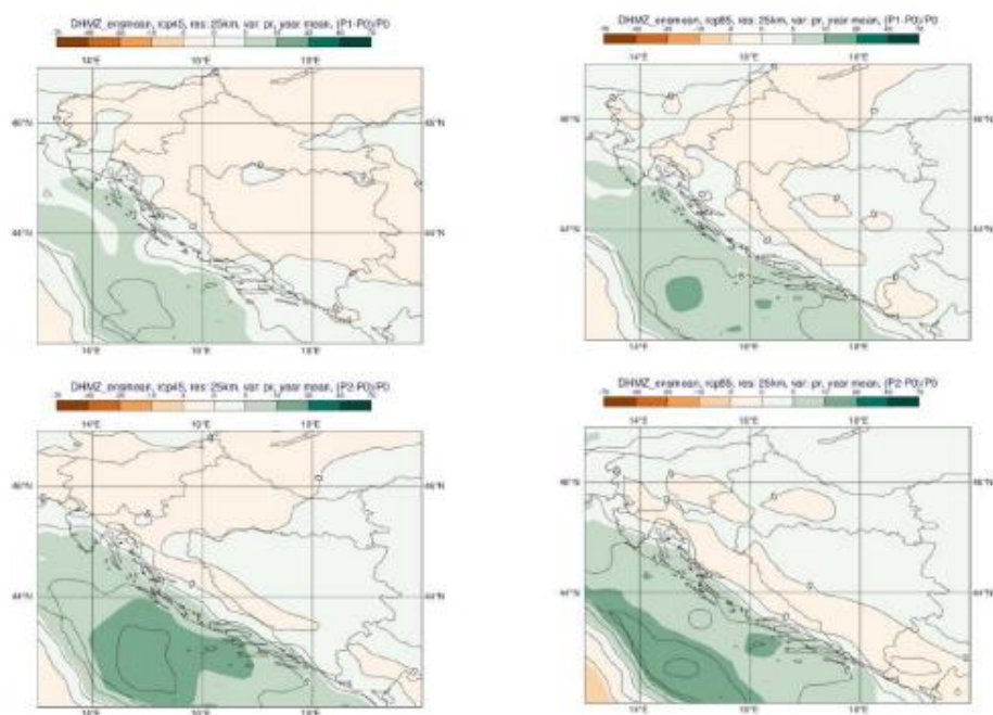
Slika 8-2 Promjena srednje godišnje ukupne količine oborine (%) u odnosu na referentno razdoblje 1971.-2000. u srednjaku ansambla iz četiri integracije RegCM modelom. Gore: za razdoblje 2011.-2040. godine; dolje: za razdoblje 2041.-2070. godine. Lijevo: scenarij RCP4.5; desno: scenarij RCP8.5.
