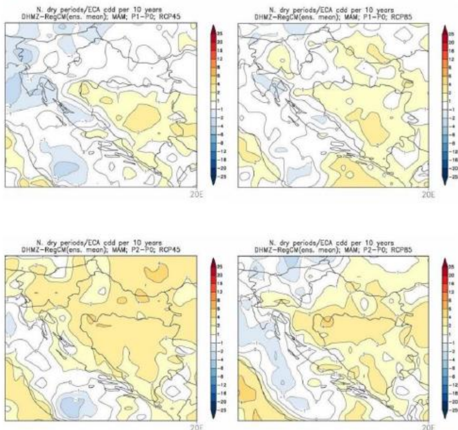
Slika 8-7 Promjena srednjeg broja sušnih razdoblja, u odnosu na referentno razdoblje 1971. – 2000. Gore: za razdoblje 2011. – 2040. godine; dolje: za razdoblje 2041. – 2070. godine; lijevo: scenarij RCP4.5; desno: scenarij RCP8.5. Mjerna jedinica: broj događaja u 10 godina. Sezona: proljeće.
