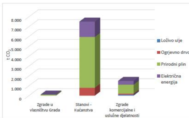
Slika 5-1 - Kontrolni inventar emisije CO 2 iz sektora zgradarstva grada Belišća prema podsektorima i energentima za 2020. godinu
