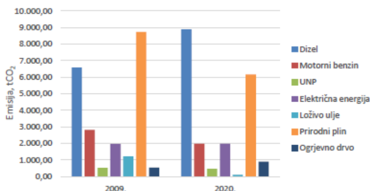
Slika 6-1 - Usporedba Referentnog i Kontrolnog inventara emisija CO 2 po energentima
