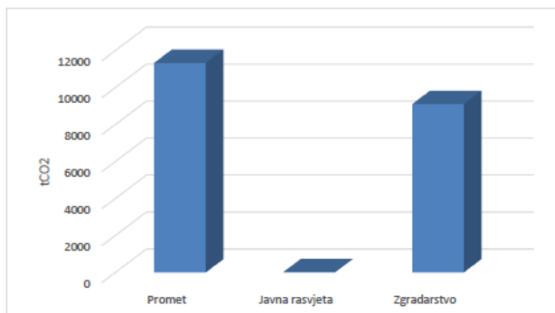
Slika 5-8 - Kontrolni inventar emisija CO 2 po sektorima u 2020. godini
